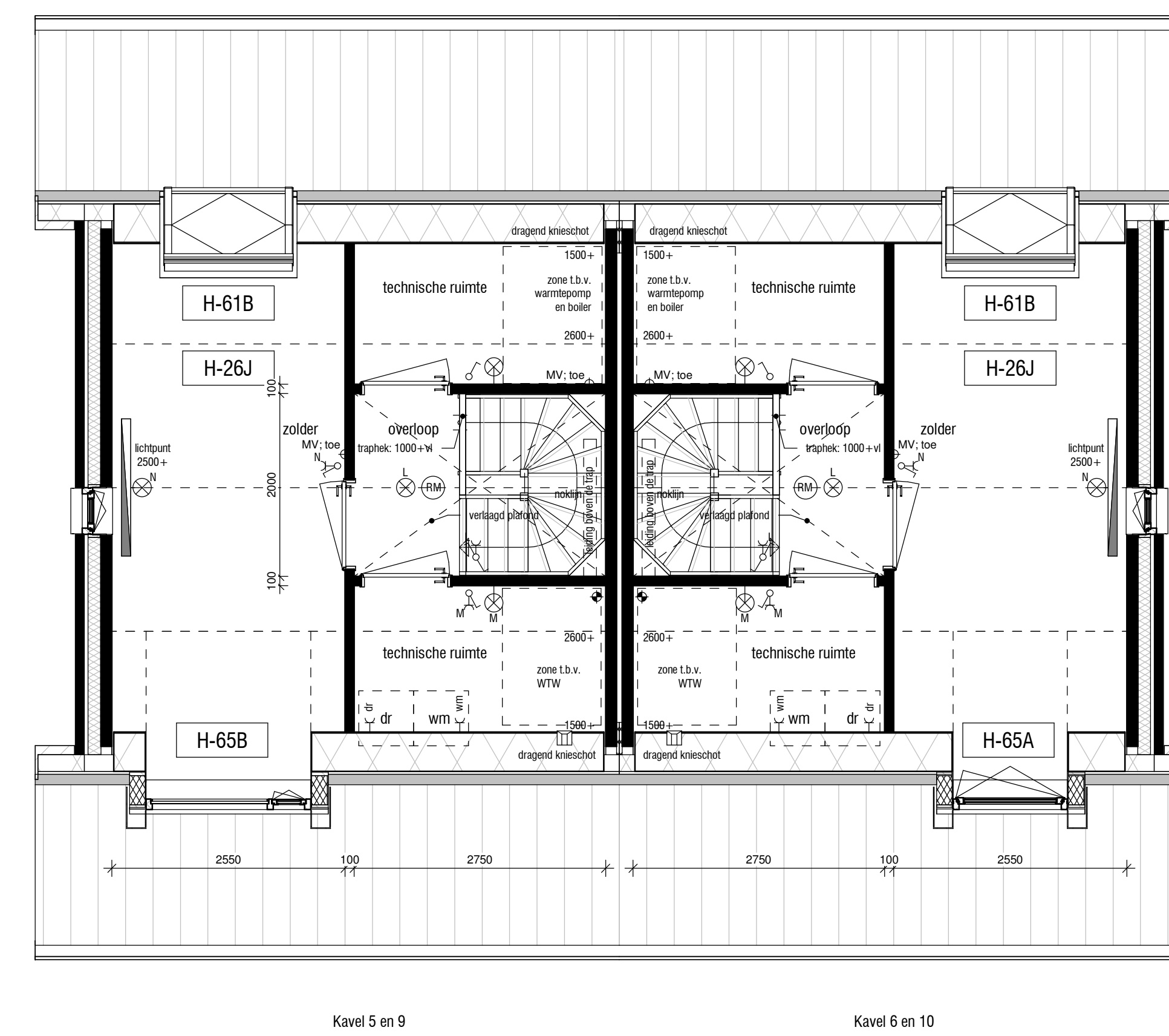
Tweede verdieping schaal 1 : 50
