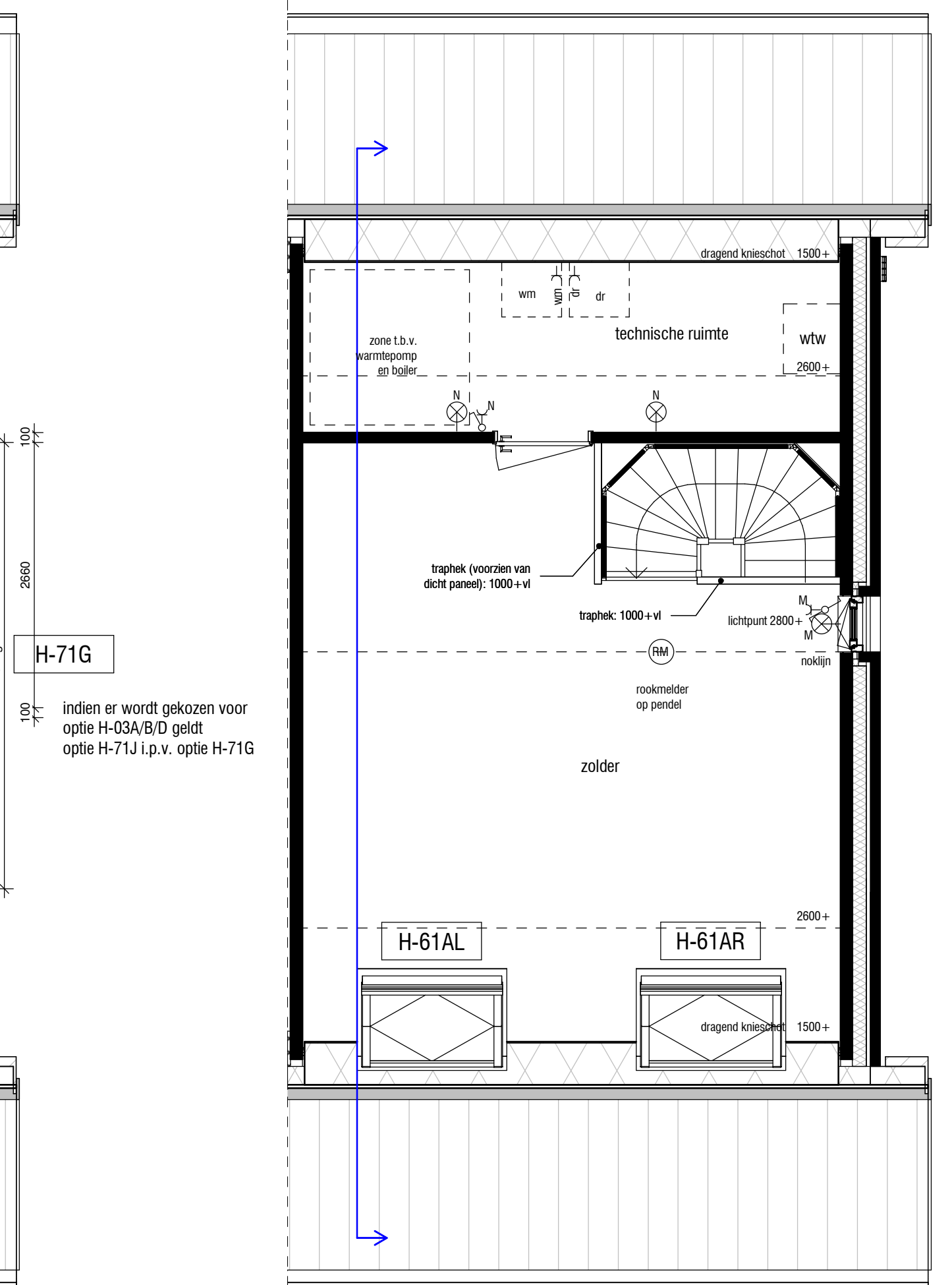
Tweede verdieping Kavel 14 en 24 schaal 1 : 50
