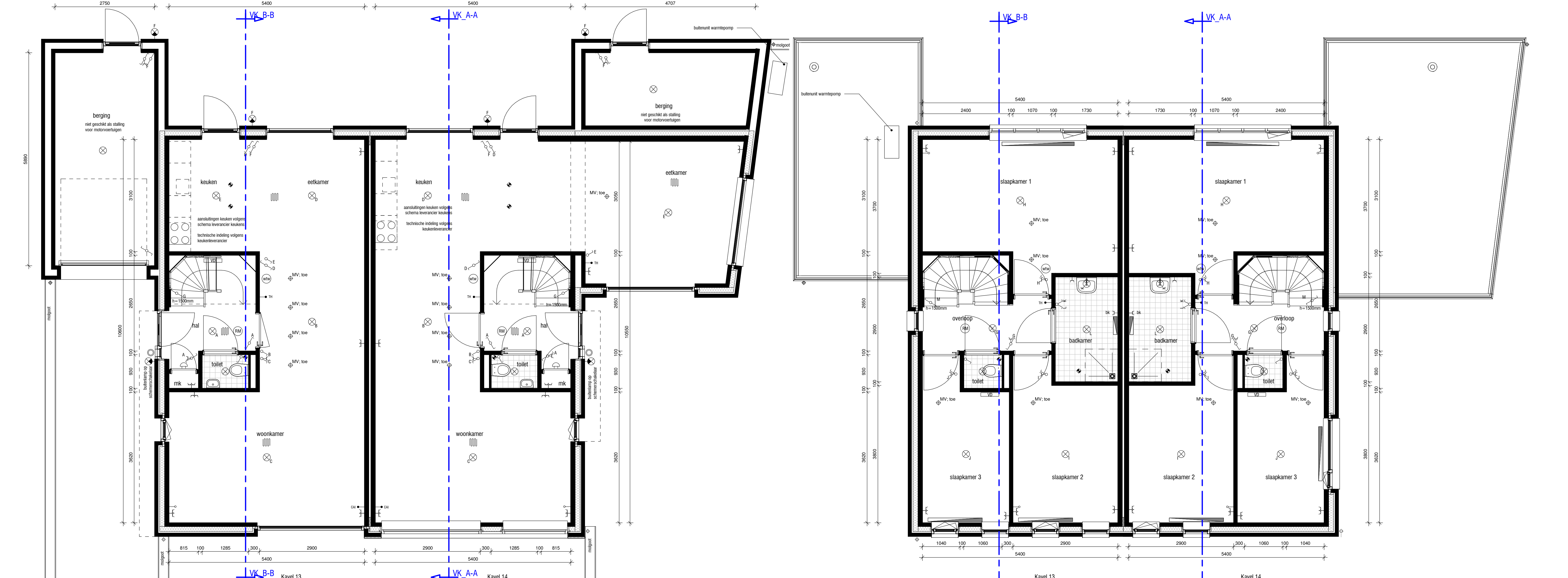
Begane grond schaal 1 : 50 Eerste verdieping schaal 1 : 50
