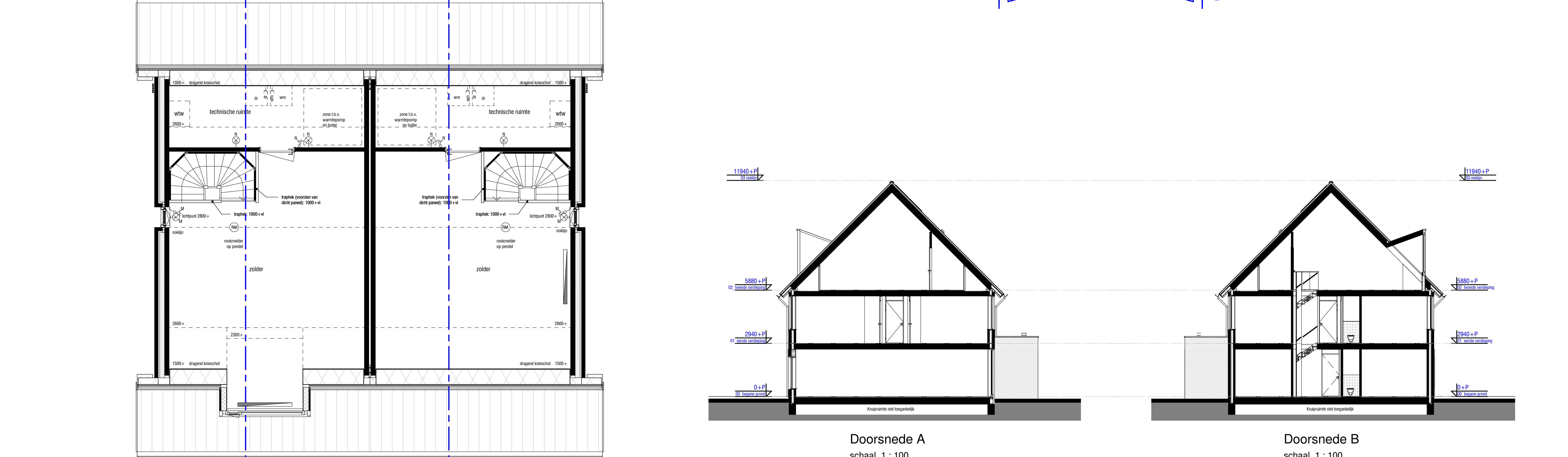
Tweede verdieping schaal 1 : 50 Doorsnede A schaal 1 : 100 Doorsnede B schaal 1 : 100
