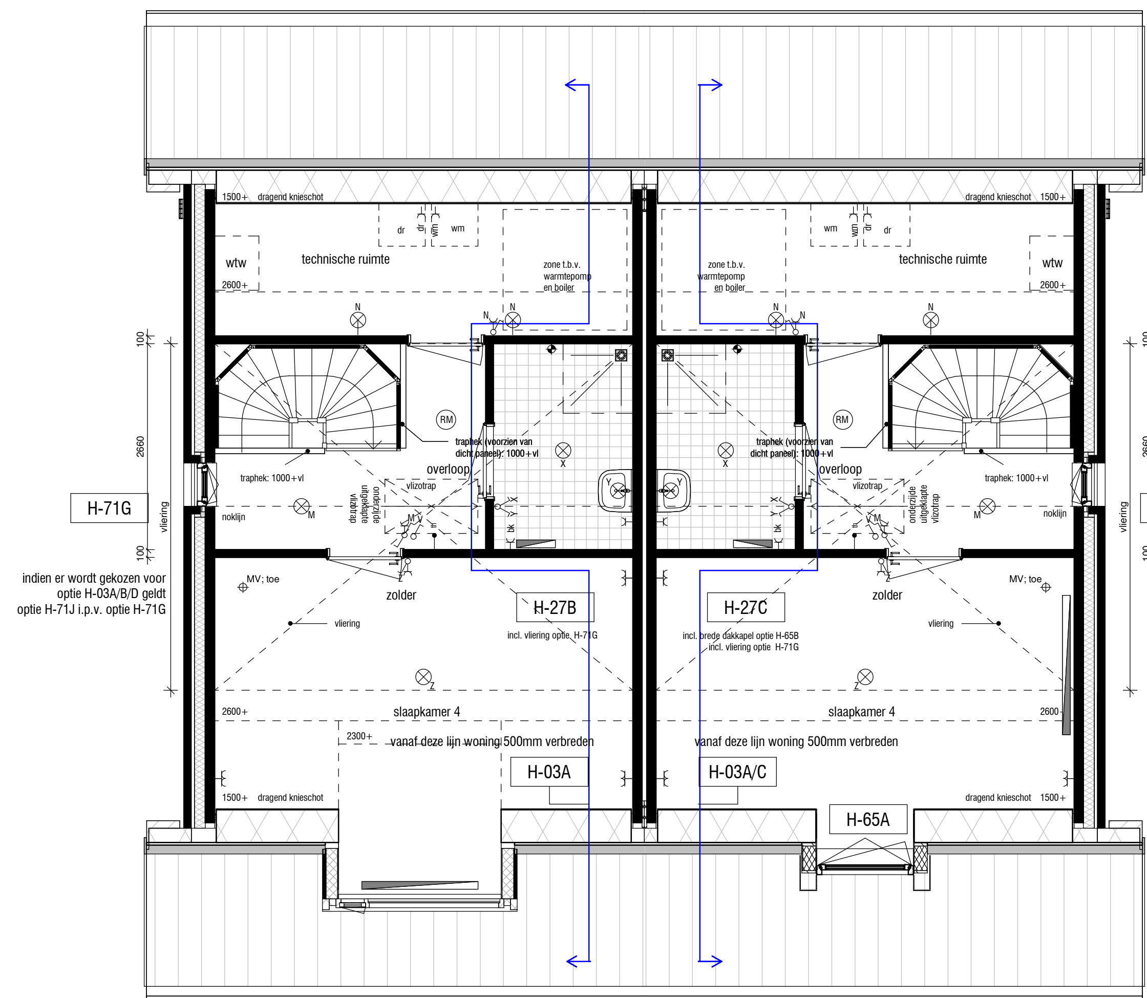
Tweede verdieping Kavel 13 en 23 schaal 1 : 50
