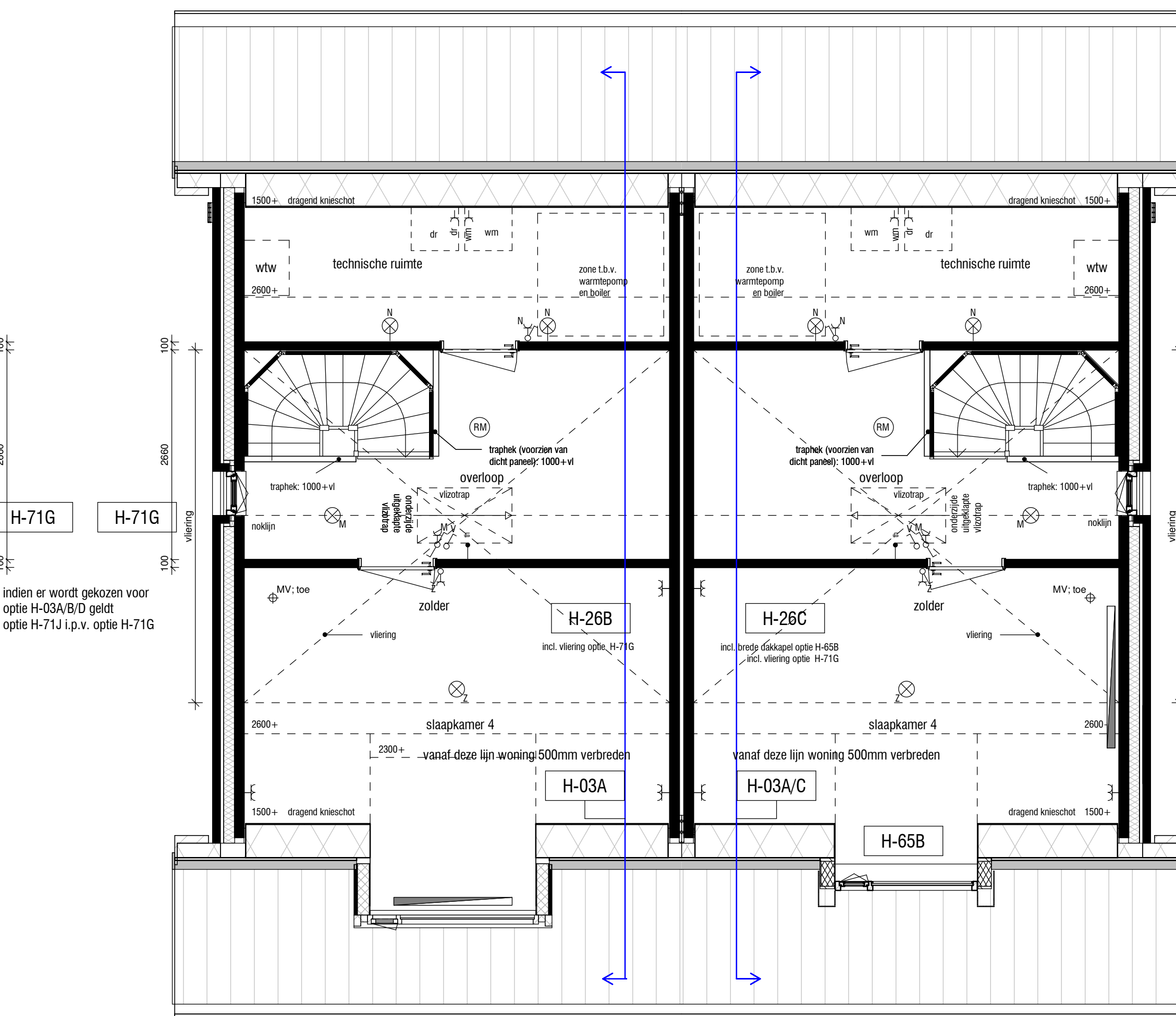
Tweede verdieping Kavel 14 en 24 schaal 1 : 50
