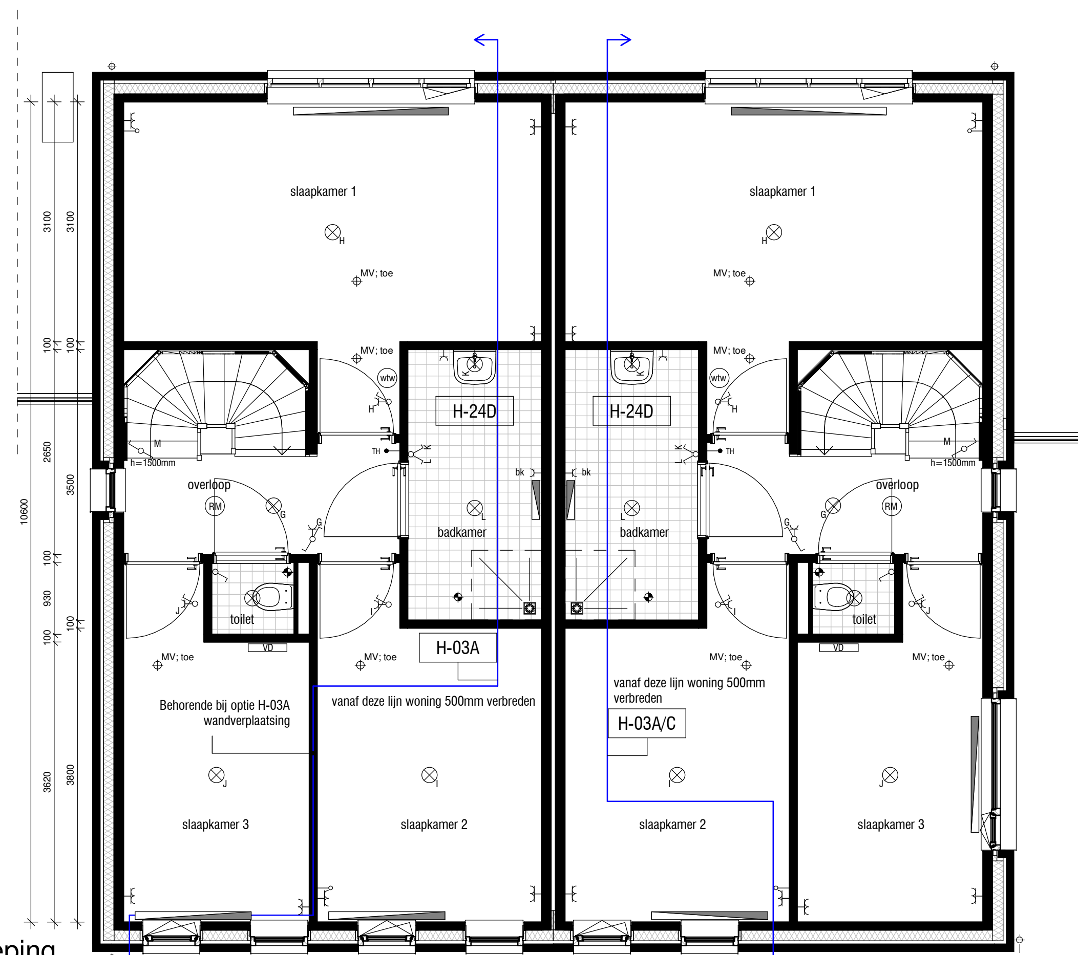
Eerste verdieping Kavel 14 en 24 schaal 1 : 50
